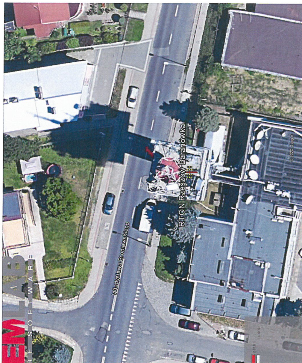
Rys. 2. Rzut poziomy rozkładu pola elektromagnetycznego anteny nowo projektowanej linii radiowej w otoczeniu RTON Rzeszów / Baranówka przewidzianej do zainstalowania na wysokości 42 m nad poziomem terenu.
